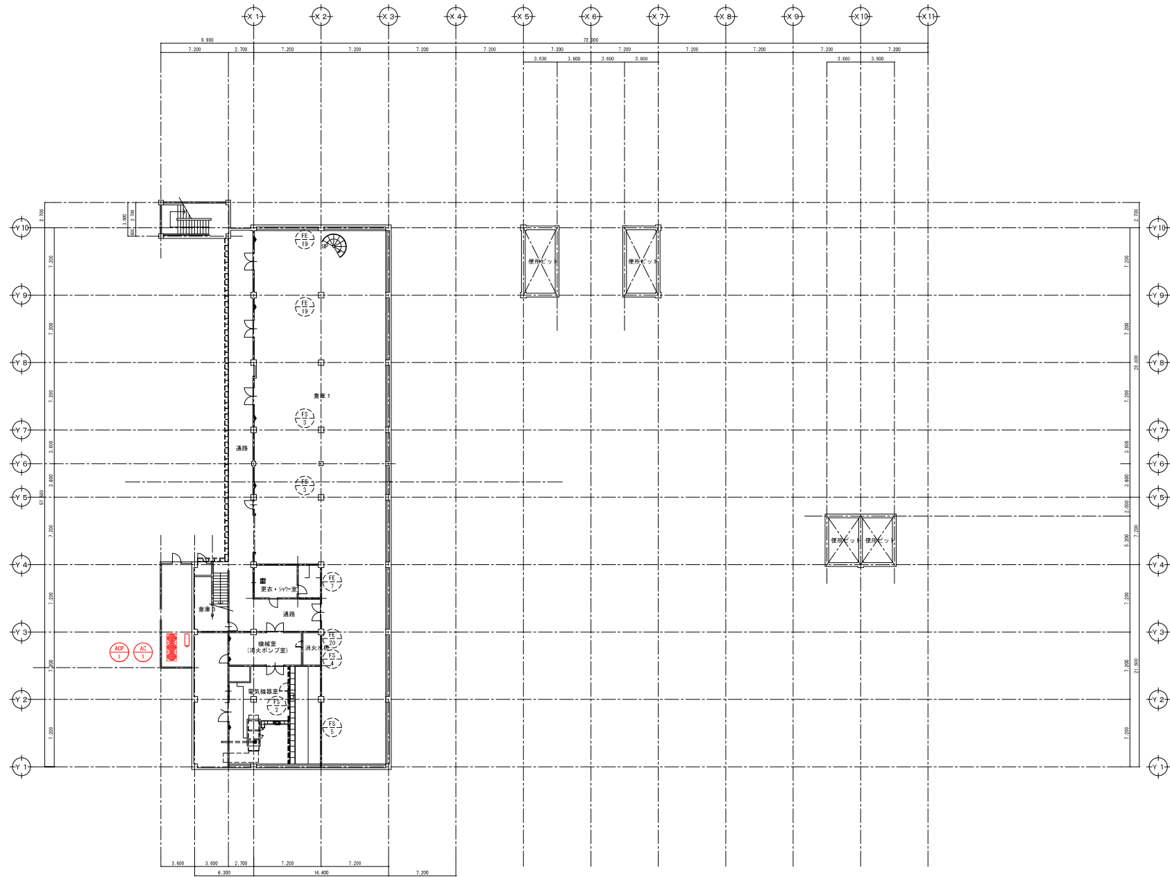
地下1階平面図 S=1:200
